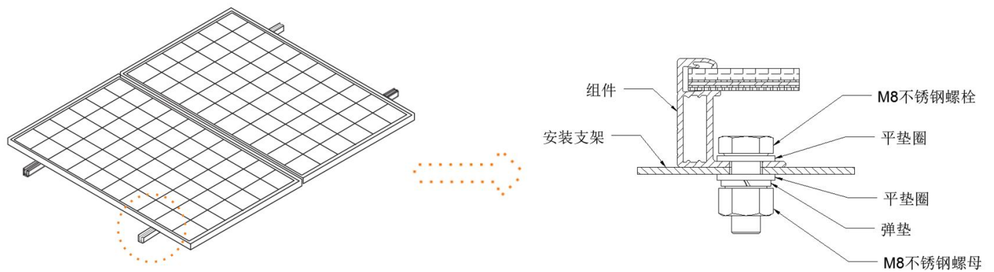
图 17 铝边框组件螺栓孔安装
