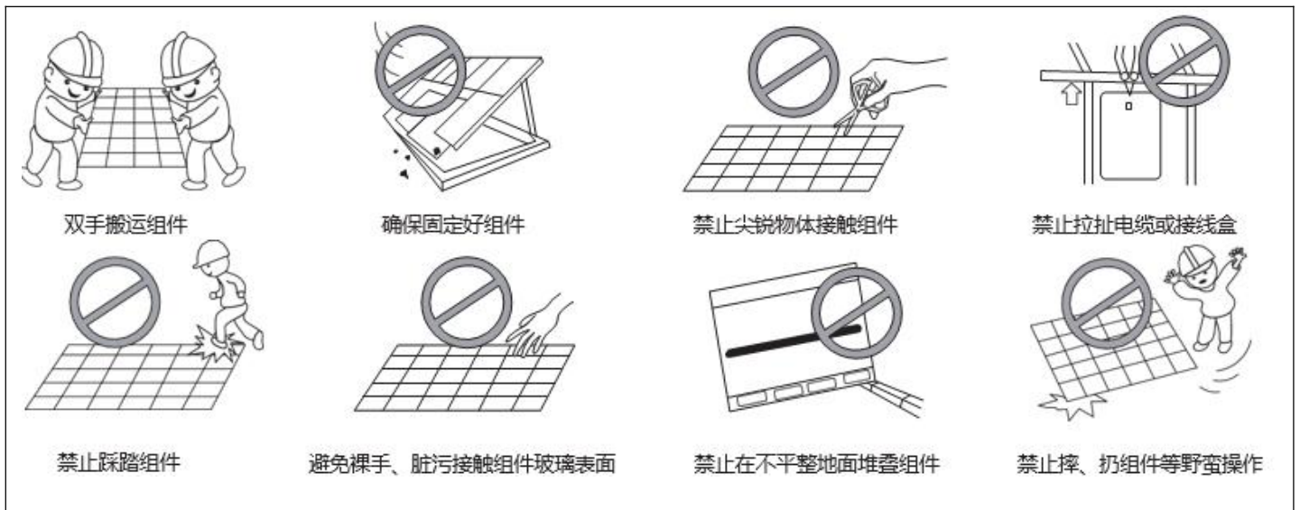
图 14 组件搬运说明
