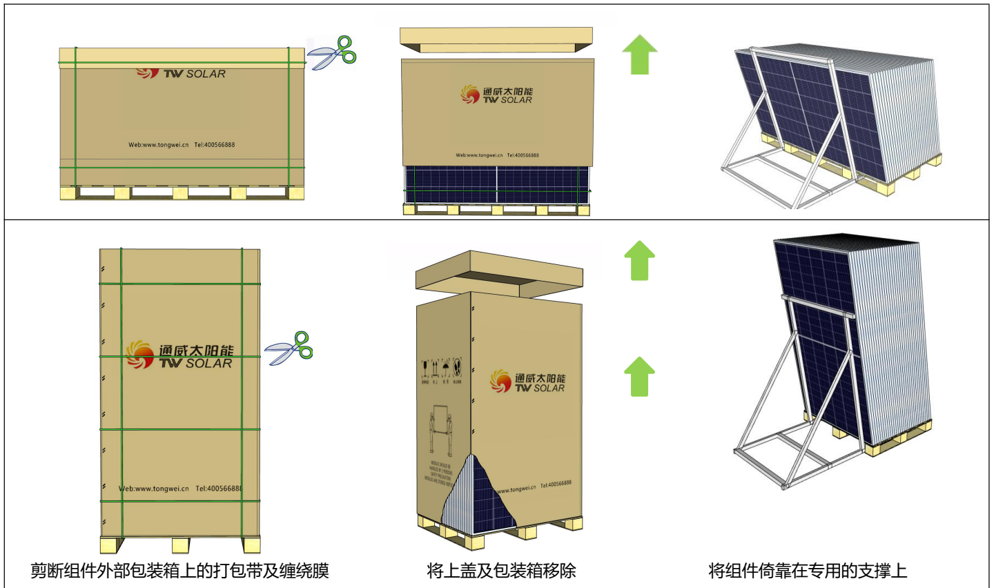
图13 组件拆箱步骤示意图
