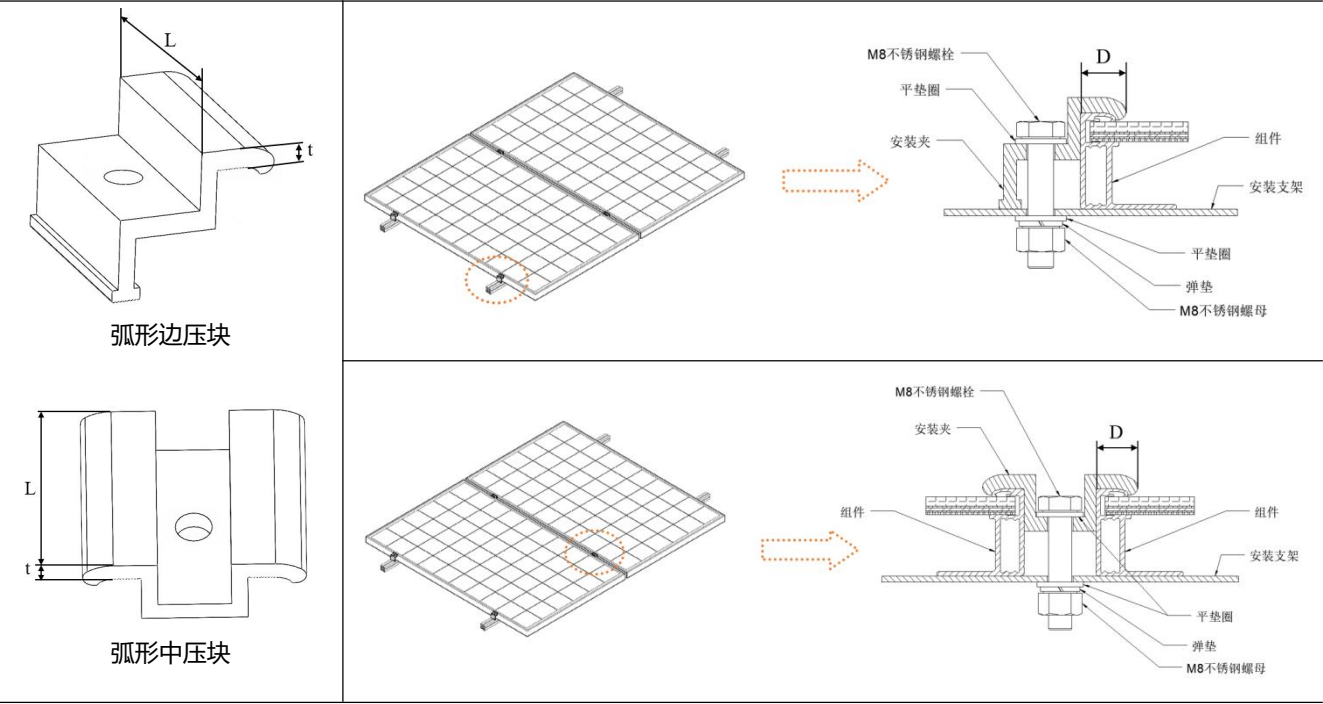
图 16 铝边框组件压块安装
