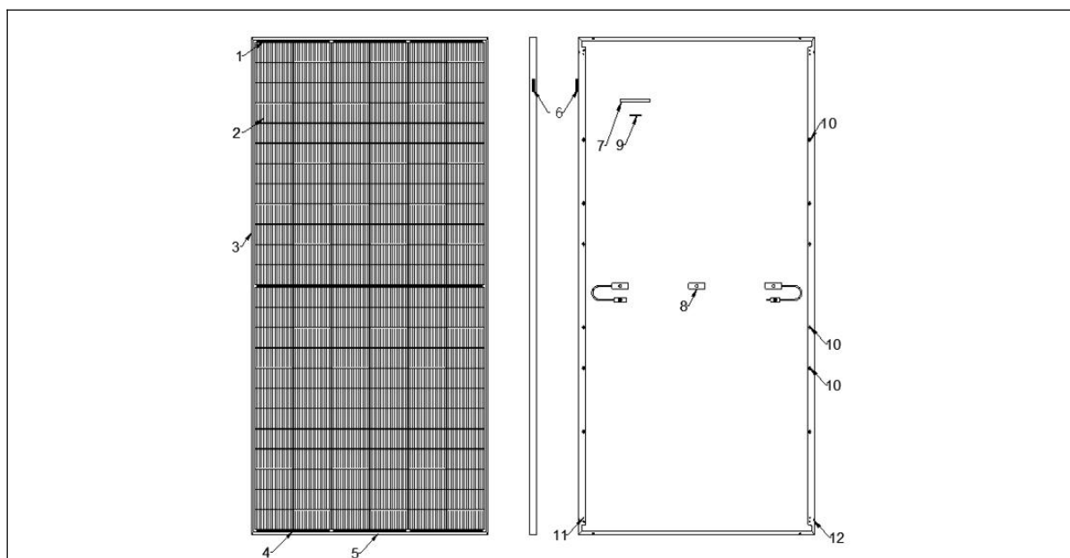
图1 单玻组件结构示意图及部件说明
