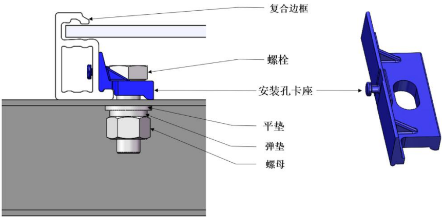
图19 复合边框组件螺栓安装
