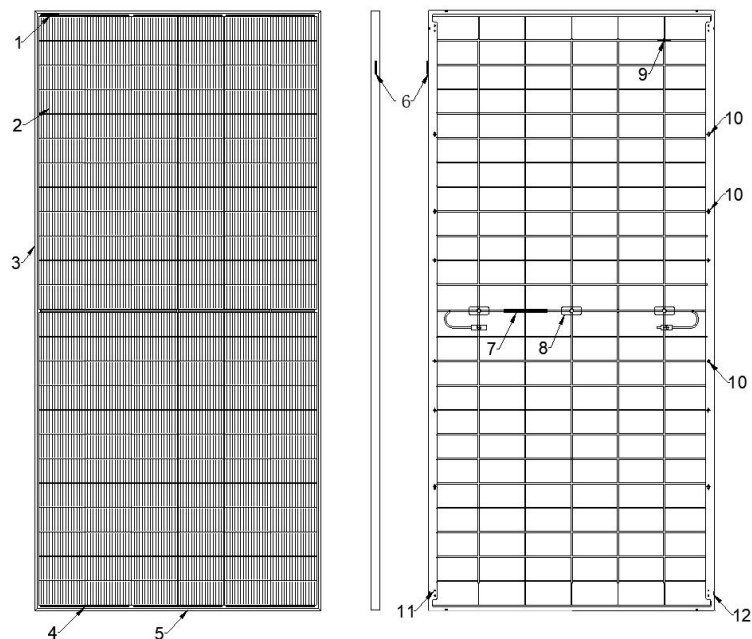
图2 双玻组件结构示意图及部件说明
