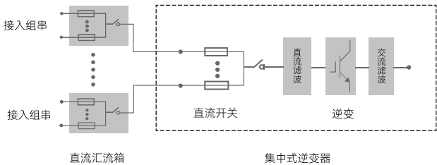
集中式逆变器系统原理图
