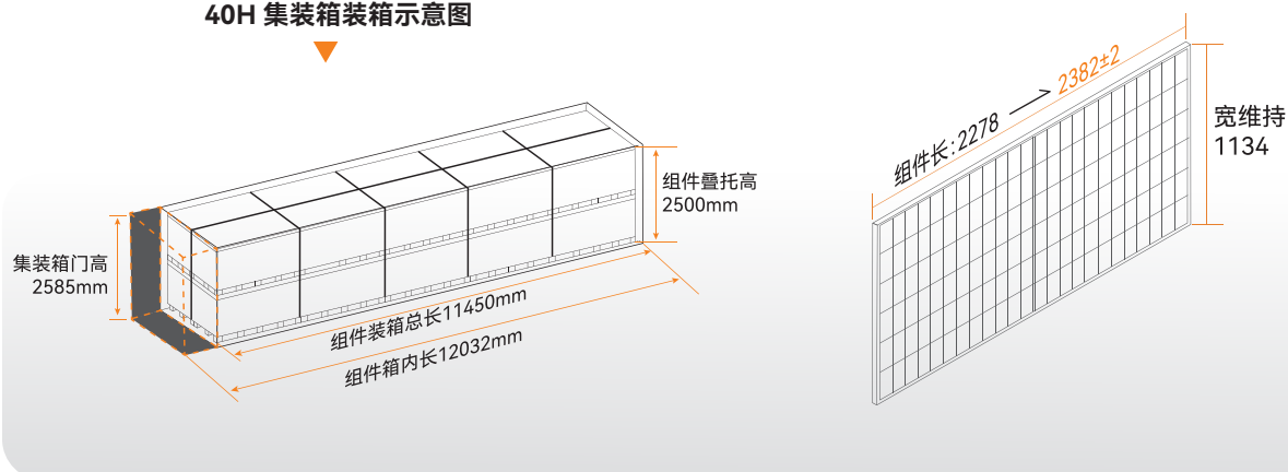
40H 集装箱装箱示意图
