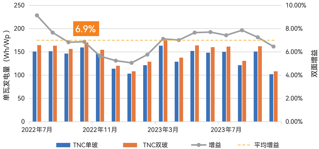
双面双玻组件实证增益
