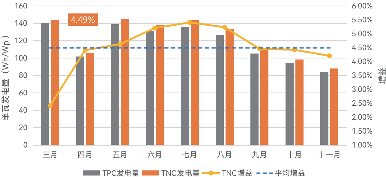
TNC与TPC组件实证对比
