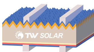
TNC 电池结构示意图
