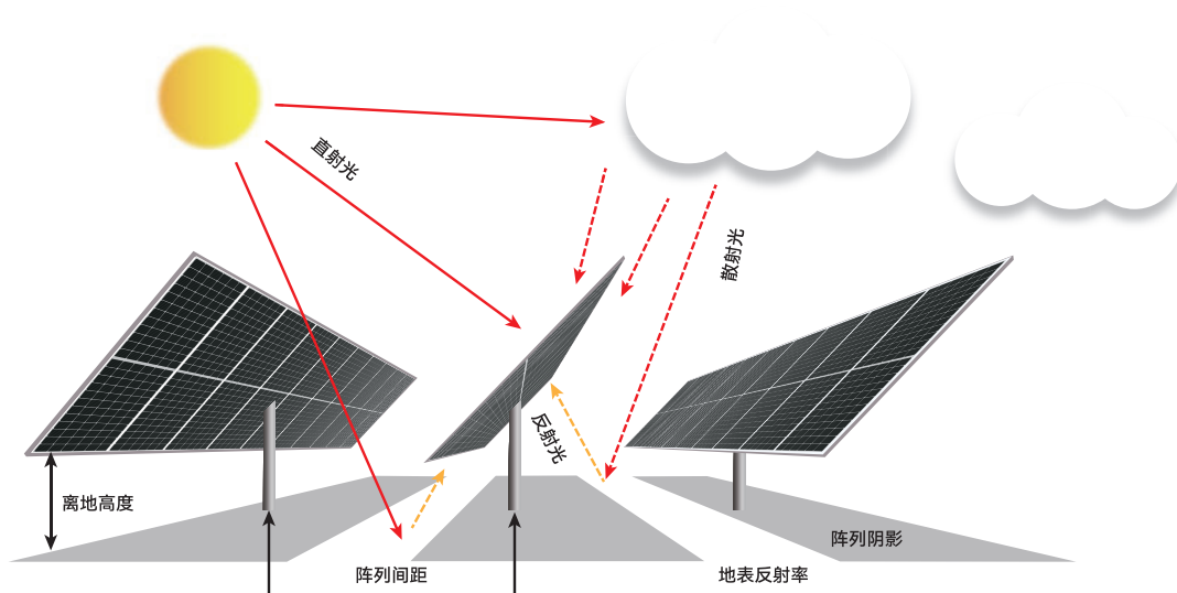
双面组件发电原理图
