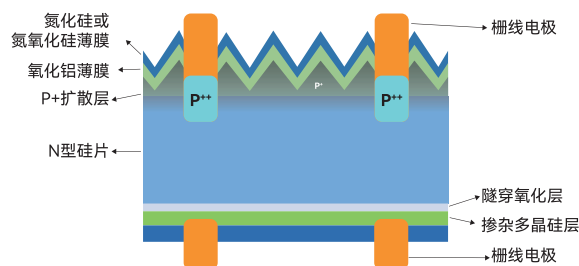
SE 激光掺杂技术示意图
