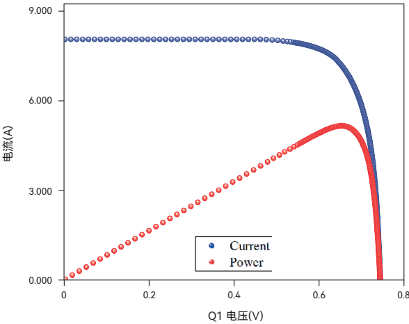
IV 曲线
