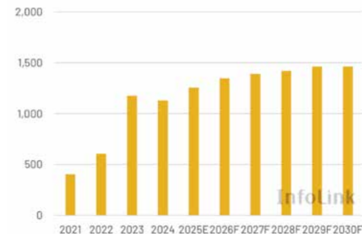
图1.2 2021-2030年全球电池片产能预测图 (单位:GW) [3]
