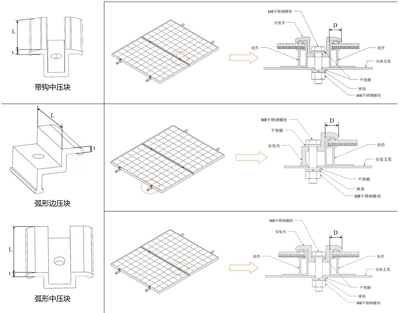
图 16 铝边框组件压块安装
