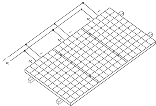
图19 并联方式
