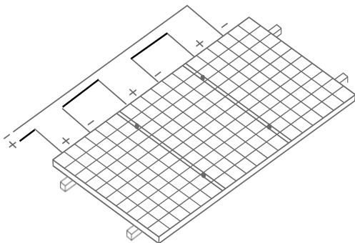
图18 串联方式
