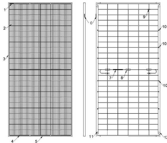
图1 双玻组件结构示意图及部件说明
